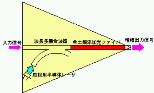
図 1.8 希土類添加光ファイバ増幅器の構成
