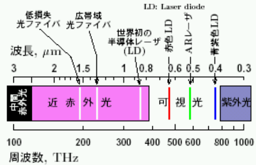
図 2.3 光通信に関わる光波の周波数と波長
